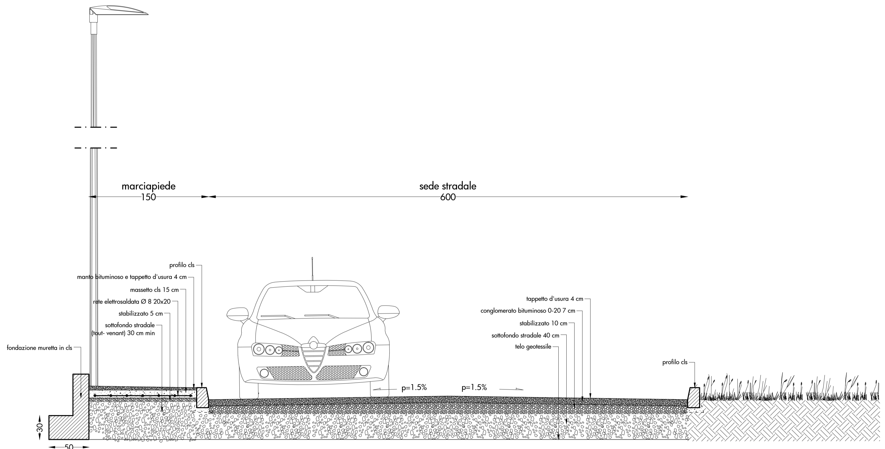
sezione a-a scala 1:25
