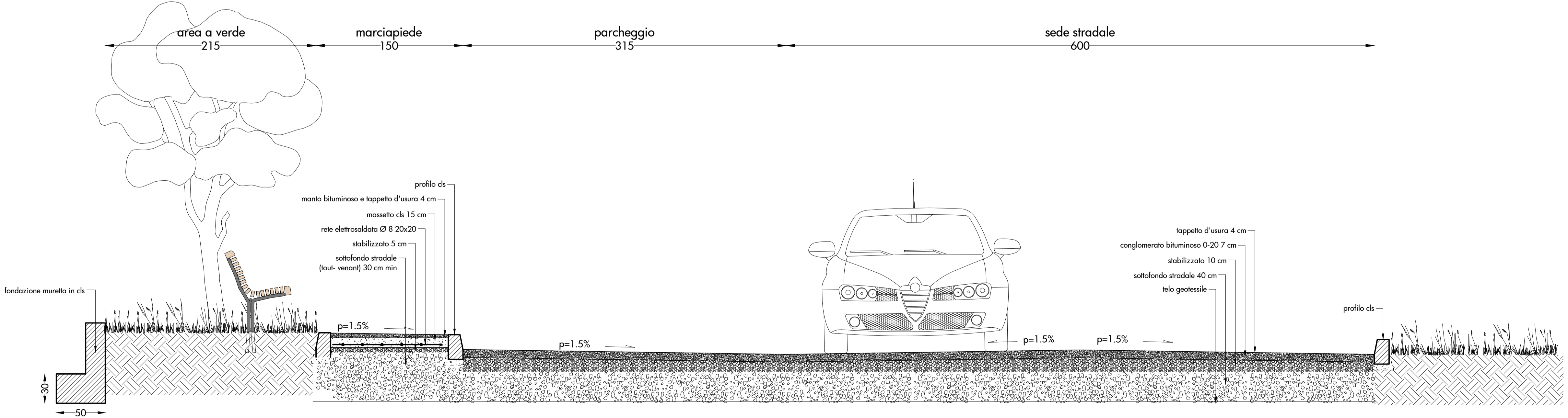
sezione b-b scala 1:25
